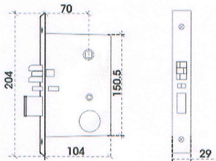
ANSI Mortise
